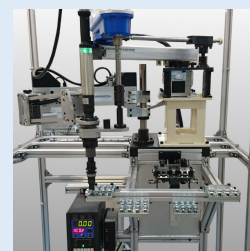
スカラロボット+トレーサアーム 自動ボルト締めユニット
